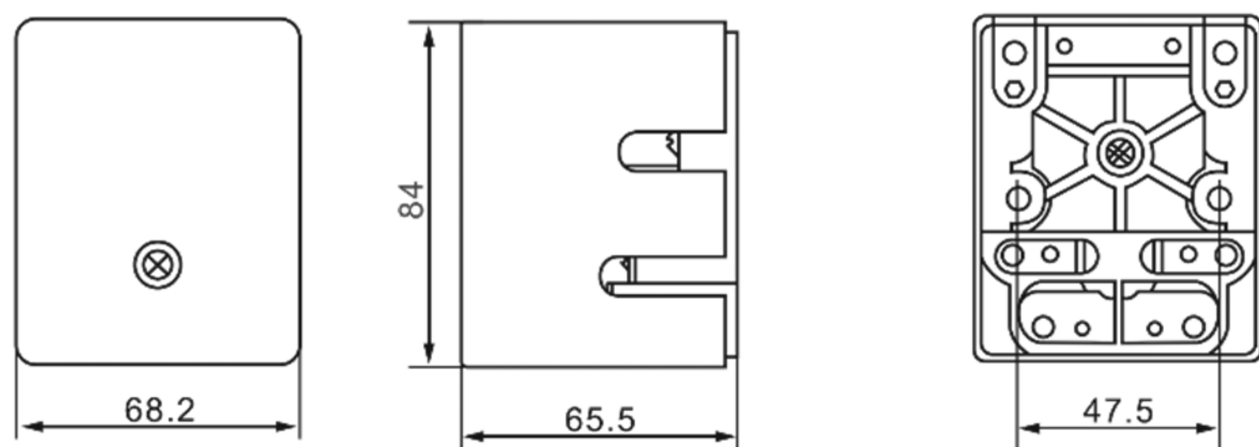
JQX-62F-2Z (Крепление на винты)
