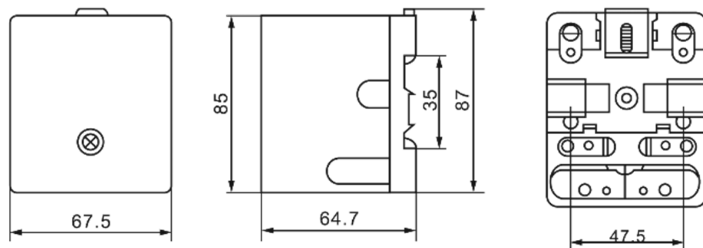
JQX-62FH-2Z (Крепление на DIN рейку)
