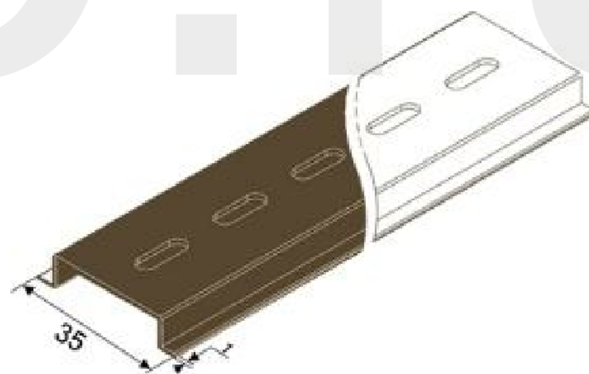
Тип DIN-рейки
