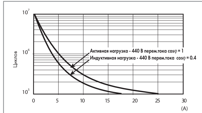
F 66 - Электрическая долговечность (АС) при номинальной нагрузке 440 В (нормально открытый контакт)
