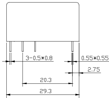
安装图
