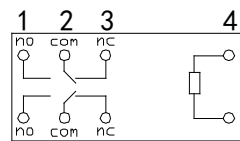
接线图
