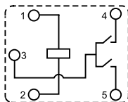
接线方法1
