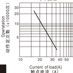
Life Expectancy 寿命曲线
