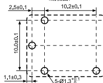
安装孔尺寸 (底视图)
