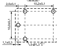
安装孔尺寸 (底视图)
